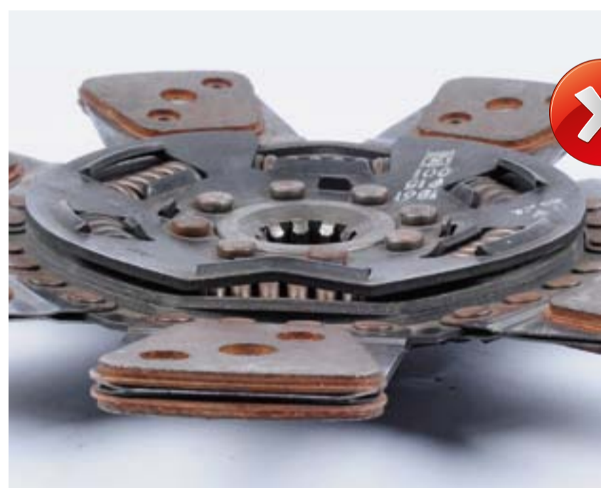
Behajlott kuplungtárcsa elferdült aggyal
